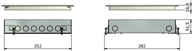
Zijaanzichten VELOX 2.0 met Slot (op deze tekening is het slot niet meegenomen)
