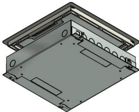
Onderaanzicht VELOX 2.0 met Slot
