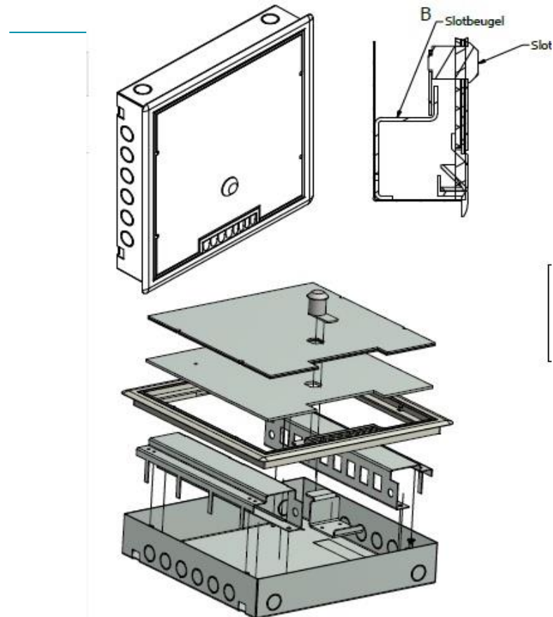
Vloerkanaal serpa
