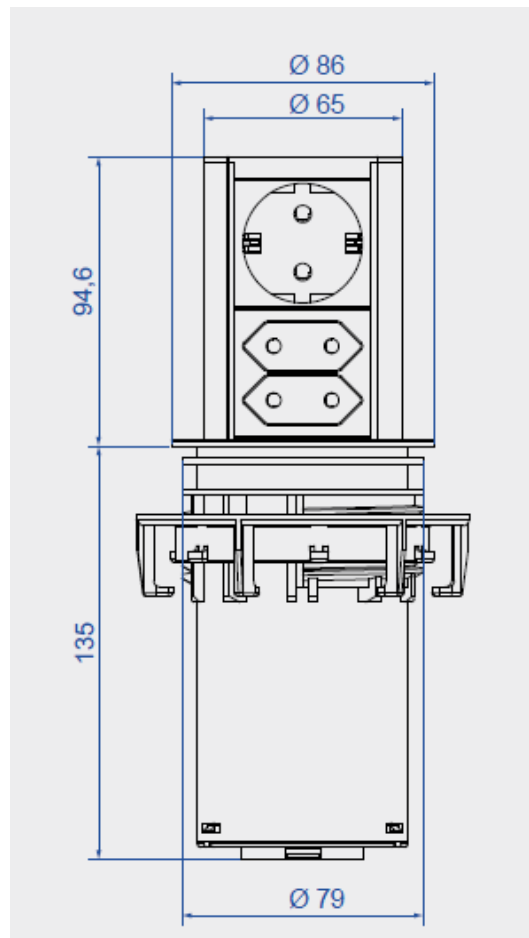
Schets met afmetingen
