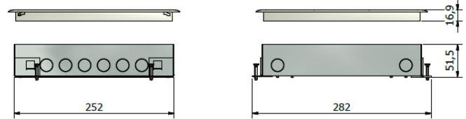
Zijaanzichten VELOX 2.0 met Kunststoff deksel
