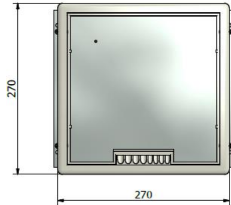
Bovenaanzicht VELOX 2.0 met Kunststoff deksel
