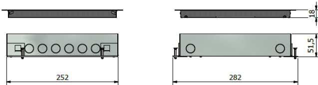
Zijaanzichten VELOX 2.0 met RVS deksel
